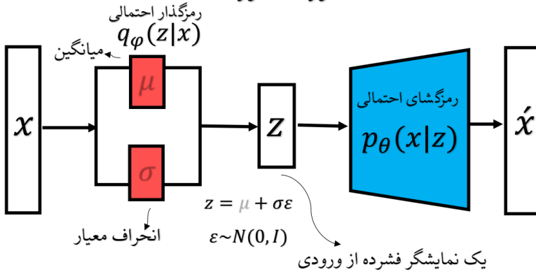
شکل ۳-۶ معماری خودرمزنگار متغیر با روند دقیق رمزگذار
