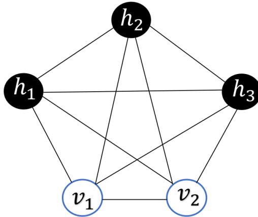
شکل ۱۲-۳ معماری یک ماشین بولتزمن با دو گره قابل رویت و ۳ گره پنهان
