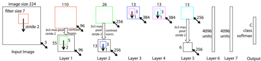
شکل ۲-۴۲ معماری AlexNet
