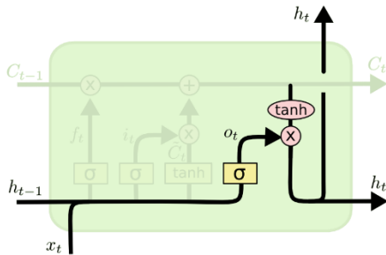
شکل ۳۰-۲ دروازه خروجی
