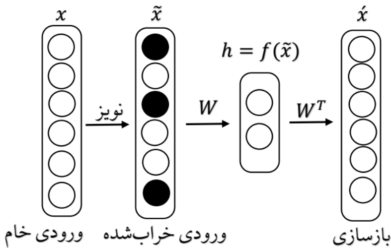
شکل ۲-۳ معماری خودرمزنگار
