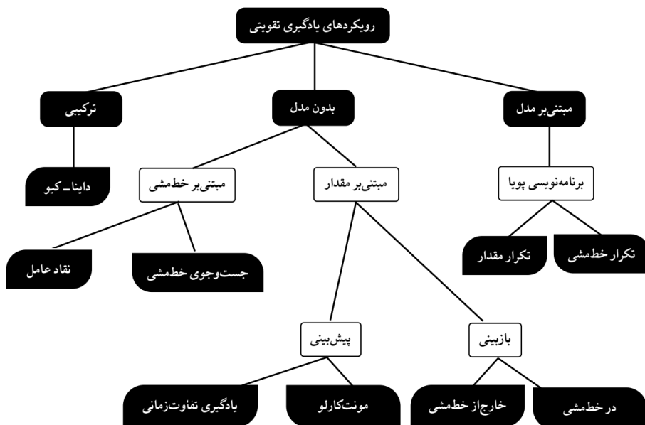
شکل ۴-۳ نحوه تقسیم‌بندی رویکردهای یادگیری تقویتی
